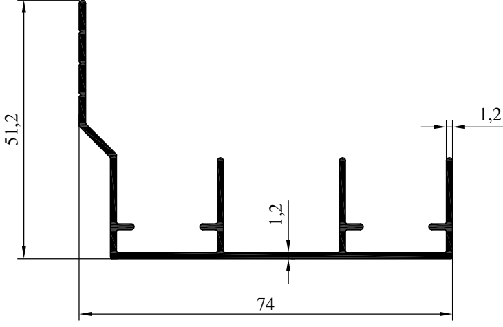
NO : 5770 AĞIRLIK : 624 gr/m
