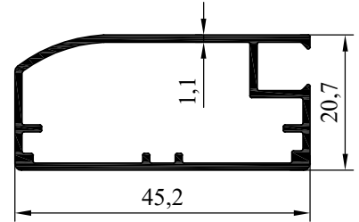
NO : 3559 AGIRLIK : 0.437 kg/m
