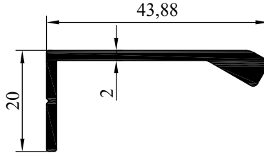
NO:7832 AĞIRLIK: 415 gr/m
