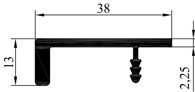
NO : 4990 AĞIRLIK : 0.397 kg/m
