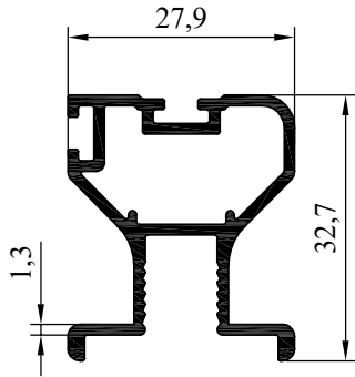
NO : 3523 AĞIRLIK : 0.507 kg/m
