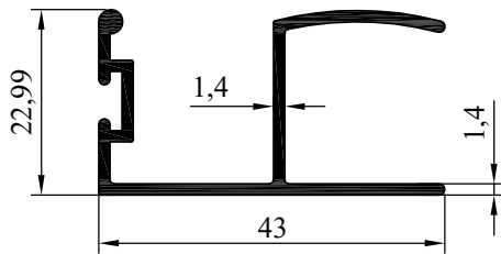
NO : 5713 AĞIRLIK : 439 gr/m
