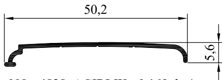
NO : 4838 AĞIRLIK : 0.169 kg/m
