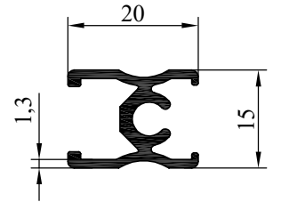
NO : 3543 AGIRLIK : 0.256 kg/m
