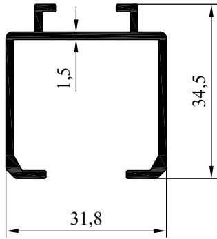
NO:7514 AĞIRLIK:478 gr/m
