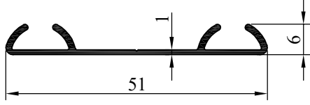
NO:6549 AĞIRLIK: 215 gr/m
