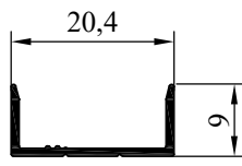
NO : 4808 AĞIRLIK : 0.096 kg/m
