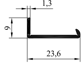
NO:7174 ĞIRLIK:116 gr/m
