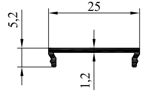
NO:6795 AĞIRLIK: 111 gr/m
