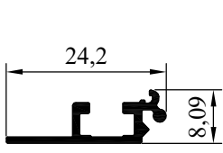
NO : 3236 AGIRLIK : 0.130 kg/m
