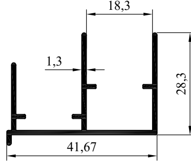
NO : 4817 AGIRLIK : 0.444 kg/m
