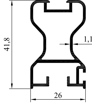
NO:6640 AĞIRLIK:518 gr/m
