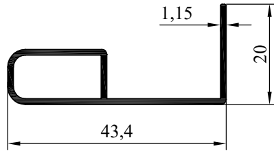
NO:6532 AĞIRLIK: 301 gr/m
