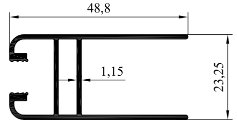
NO : 3673 AGIRLIK : 0.515 kg/m
