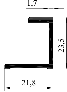
NO:6944 AĞIRLIK: 257 gr/m
