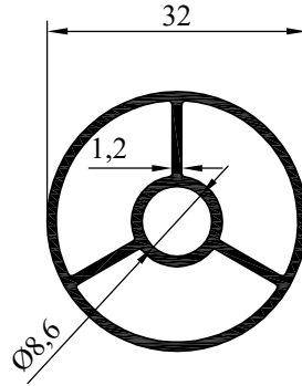
NO : 3539 AGIRLIK : 0.489 kg/m
