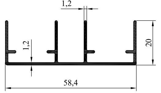
NO : 5642 AĞIRLIK: 470 gr/m
