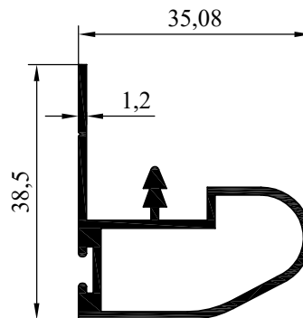
NO : 1590 AĞIRLIK : 0.472 kg/m
