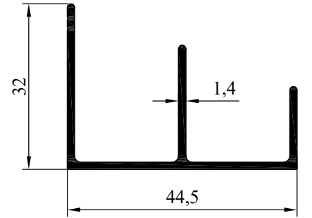
NO:7767 AĞIRLIK: 427 gr/m
