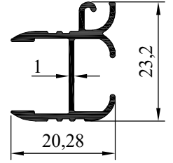
NO : 4837 AGIRLIK : 0.239 kg/m
