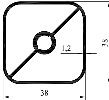
NO : 6289 AĞIRLIK : 679 gr/m
