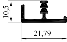
NO : 3837 AGIRLIK : 0.195 kg/m
