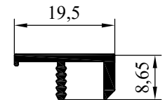
NO : 5236 AĞIRLIK : 0.150 kg/m
