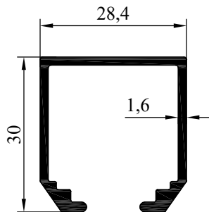
NO : 3391 AĞIRLIK : 0.446 kg/m
