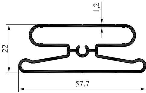
NO:6620 AĞIRLIK:733 gr/m
