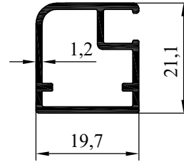
NO:7495 AĞIRLIK: 286 gr/m
