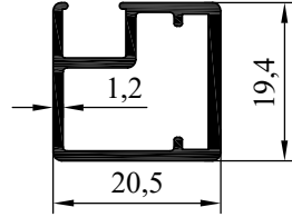
NO : 3620 AĞIRLIK : 0.290 kg/m
