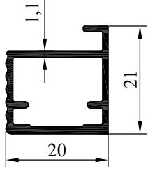
NO : 4519 AĞIRLIK : 0.270 kg/m
