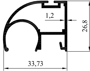
NO:6755 AĞIRLIK:463 gr/m
