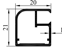
NO : 3631 AĞIRLIK : 0.257 kg/m
