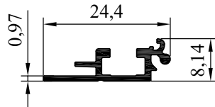
NO : 3288 AGIRLIK : 0.135 kg/m
