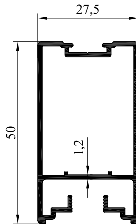
NO:6835 AĞIRLIK: 575 gr/m
