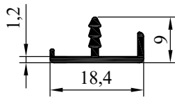
NO : 3579 AGIRLIK : 0.114 kg/m
