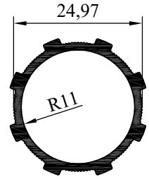
N:6659 AĞIRLIK: 376.7 gr/m
