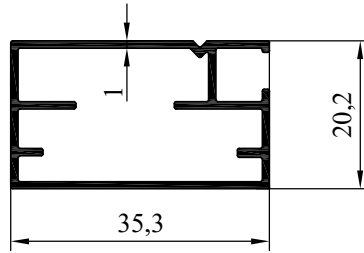
NO : 3775 AGIRLIK : 0.372 kg/m
