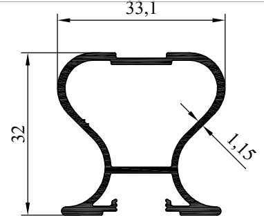
NO : 4411 AĞIRLIK : 0.474 kg/m
