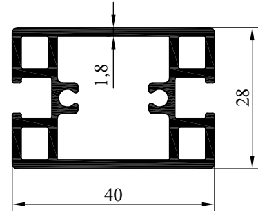
NO : 3663 AĞIRLIK : 0.954 kg/m
