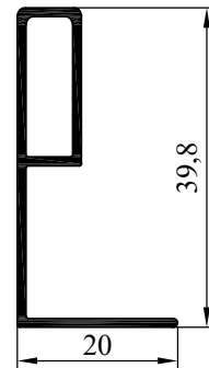
NO:10909 AĞIRLIK: 0.267 gr/m
