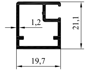
NO:7496 AĞIRLIK:289 gr/m
