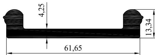
NO:7776 AĞIRLIK:1080 gr/m
