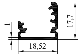
NO : 4951 AĞIRLIK : 0.181 kg/m
