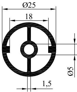
NO : 5479 AĞIRLIK : 520 gr/m
