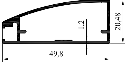
NO : 2021 AGIRLIK : 0.494 kg/m
