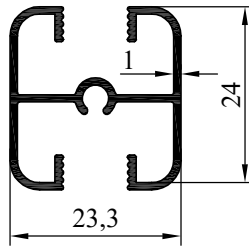
NO:6544 AĞIRLIK:304 gr/m
