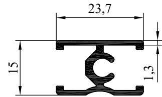
NO:6751 AĞIRLIK: 295 gr/m
