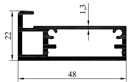
NO : 3572 AĞIRLIK : 0.715 kg/m
