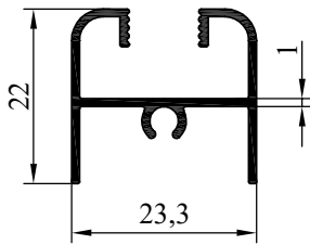
NO:6543 AĞIRLIK:247 gr/m
