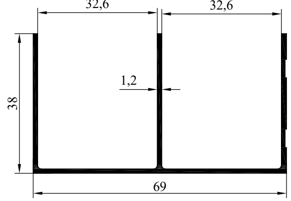
NO : 3669 AGIRLIK : 0.592 kg/m
