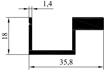
NO:6624 AĞIRLIK: 461 gr/m
