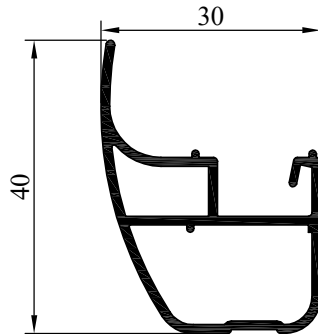
NO:6750 AĞIRLIK:448 gr/m
