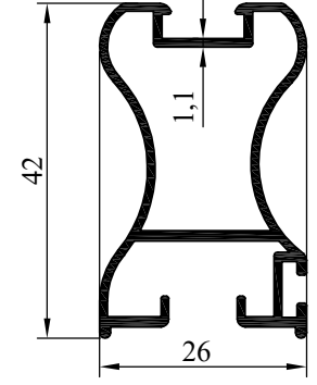
NO:6668 AĞIRLIK: 483 gr/m
