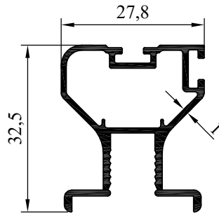
NO :3670 AĞIRLIK : 0.425 kg/m
