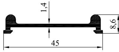
NO:8107 AĞIRLIK: 303 gr/m
