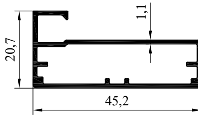
NO : 3558 AGIRLIK : 0.427 kg/m
