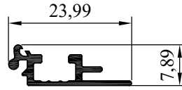
NO:7722 AĞIRLIK: 130 gr/m
