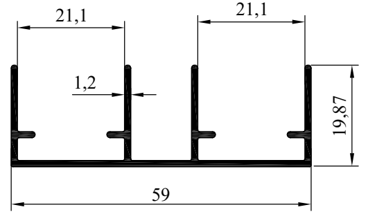
NO : 3399 AĞIRLIK : 0.477 kg/m
