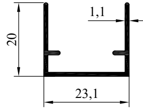
NO:6551 AĞIRLIK: 200 gr/m
