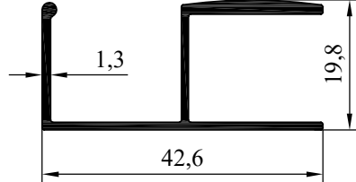
NO:6647 AĞIRLIK:367 gr/m
