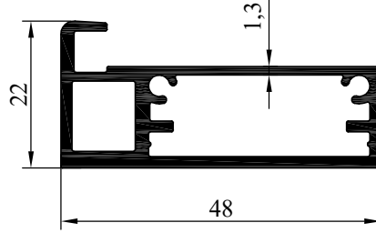
NO : 3572 AGIRLIK : 0.715 kg/m
