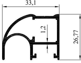
NO : 4451 AGIRLIK : 0.447 kg/m
