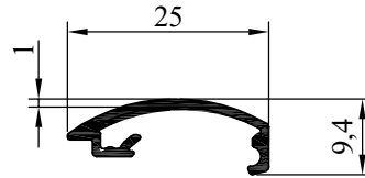
NO : 5514 AĞIRLIK : 124 gr/m
