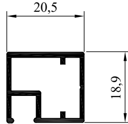
NO:7971 AĞIRLIK:276 gr/m
