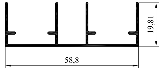
NO:6652 AĞIRLIK: 416 gr/m
