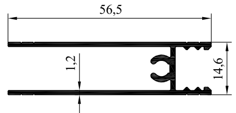
NO : 3475 AGIRLIK : 0.474 kg/m
