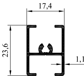
NO: 8062 AĞIRLIK: 257 gr/m
