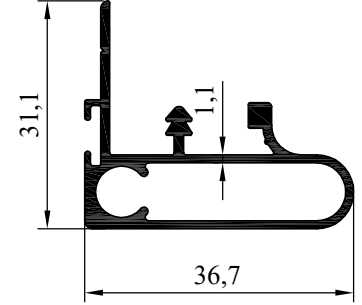
NO : 4818 AĞIRLIK : 0.457 kg/m
