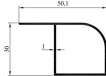
NO : 4802 AGIRLIK : 0.351 kg/m
