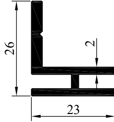
NO: 7896 AĞIRLIK:416 gr/m
