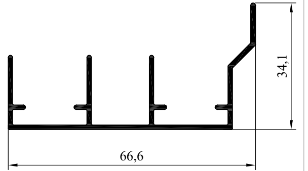
NO:7958 AĞIRLIK: 577 gr/m
