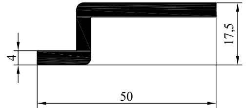
NO : 4992 AĞIRLIK : 0.682 kg/m
