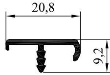
NO : 6204 AĞIRLIK : 134 gr/m
