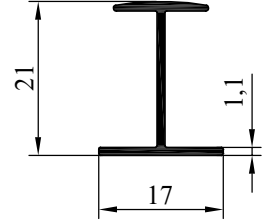
NO:6661 AĞIRLIK:146 gr/m
