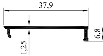
NO:6598 AĞIRLIK:155 gr/m
