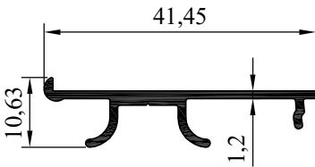
NO:6600 AĞIRLIK:242 gr/m
