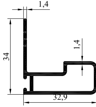
NO : 5736 AĞIRLIK : 432 gr/m
