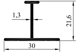
NO:6537 AĞIRLIK:198 gr/m
