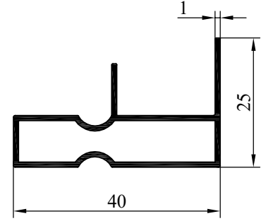
NO:6535 AĞIRLIK: 335 gr/m
