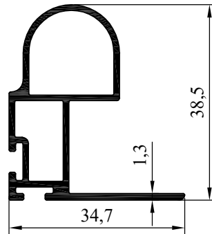
NO : 3406 AGIRLIK : 0.477 kg/m
