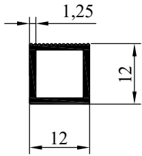
NO:7220 AĞIRLIK:142 gr/m
