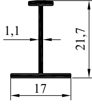
NO: 7906 AĞIRLIK: 136 gr/m
