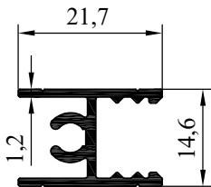
NO : 3472 AGIRLIK : 0.249 kg/m
