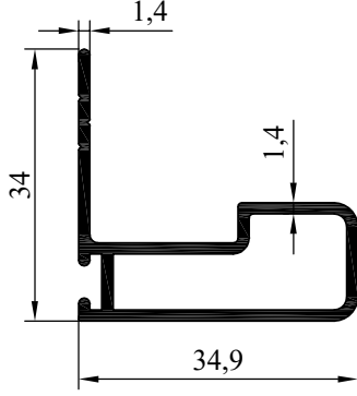
NO : 5735 AĞIRLIK : 447 gr/m
