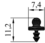
NO : 3395 AGIRLIK : 0.098 kg/m
