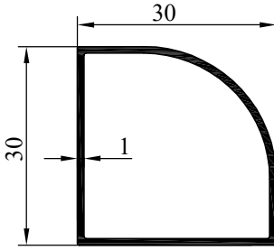
NO : 3458 AGIRLIK : 0.290 kg/m
