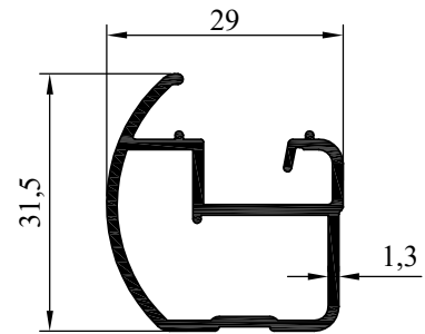
NO : 3542 AGIRLIK : 0.420 kg/m
