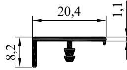
NO:6666 AĞIRLIK:113.4 gr/m
