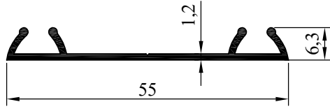
NO:6646 AĞIRLIK:255 gr/m
