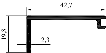
NO:6451 AĞIRLIK:397 gr/m
