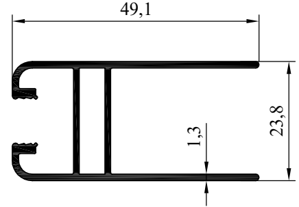
NO : 3520 AGIRLIK : 0.544 kg/m
