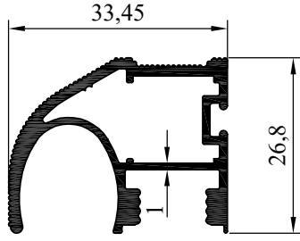
NO : 5731 AĞIRLIK : 535 gr/m
