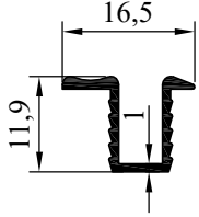
NO:6664 AĞIRLIK:108 gr/m
