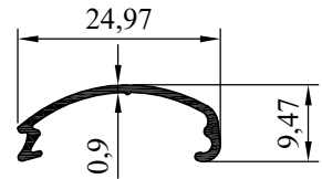
NO:7721 AĞIRLIK: 103 gr/m
