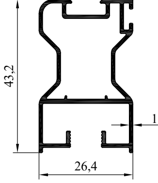
NO:6541 AĞIRLIK: 510 gr/m
