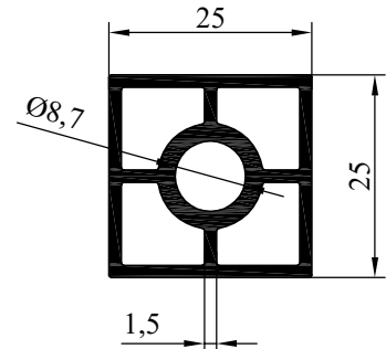
NO : 4033 AĞIRLIK : 0.652 kg/m
