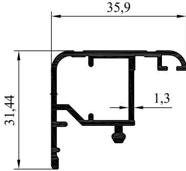
NO : 5027 AGIRLIK : 0.470 kg/m
