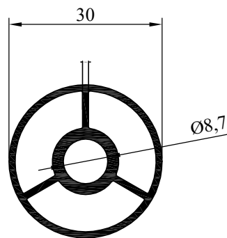
NO : 3539 AGIRLIK : 0.489 kg/m
