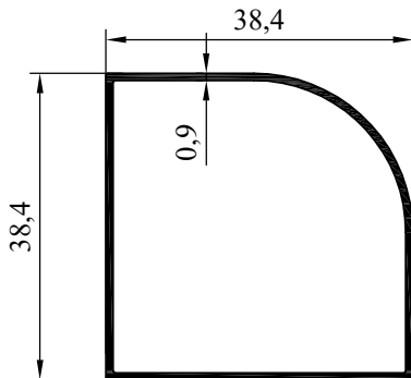
NO:6699 AĞIRLIK: 344 gr/m
