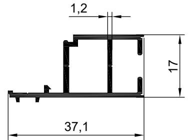
NO : 1938 AGIRLIK : 0.334 kg/m
