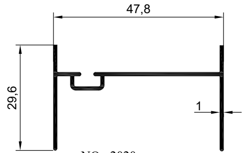
NO : 2020 AGIRLIK : 0.312 kg/m
