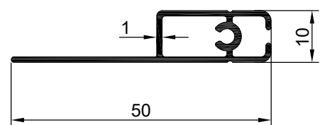
NO : 1791 AGIRLIK : 0.282 kg/m
