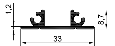
NO:7387 AĞIRLIK:232 gr/m
