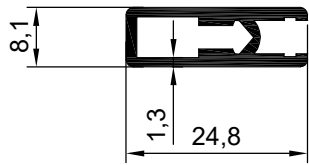
NO : 1968 AGIRLIK : 0.266 kg/m
