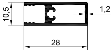
NO : 2018 AGIRLIK : 0.275 kg/m
