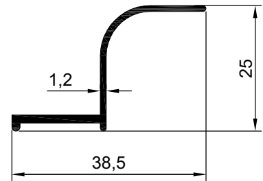
NO:2458 AGIRLIK : 0.213 kg/m
