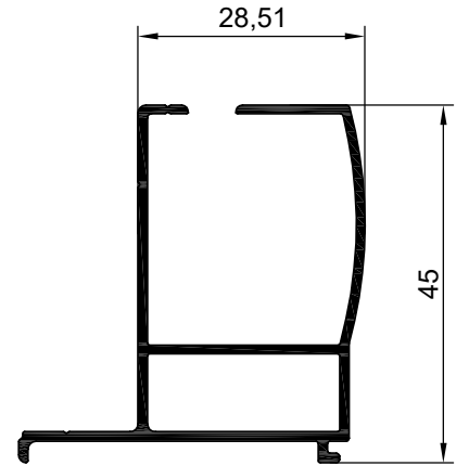
NO:7846 AĞIRLIK: 540 gr/m
