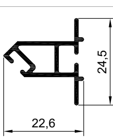
NO : 1986 AGIRLIK : 0.240 kg/m
