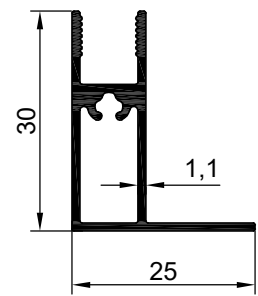
NO:7663 AĞIRLIK: 316 gr/m
