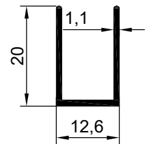
NO : 2012 AGIRLIK : 0.152 kg/m
