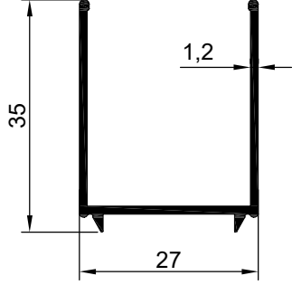
NO : 2357 AGIRLIK : 0.309 kg/m
