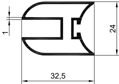
NO : 2469 AGIRLIK : 0.412 kg/m
