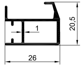
NO : 1596 AGIRLIK : 0.292 kg/m
