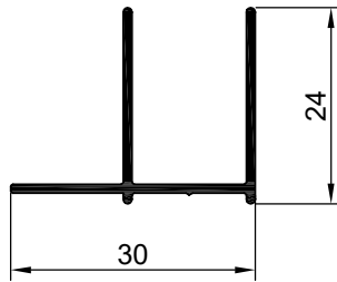
NO:7443 AĞIRLIK: 224 gr/m
