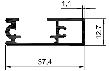
NO : 1871 AGIRLIK : 0.374 kg/m
