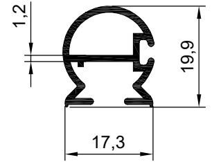
NO : 1866 AGIRLIK : 0.264 kg/m
