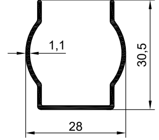
NO:6481 AĞIRLIK: 247 gr/m
