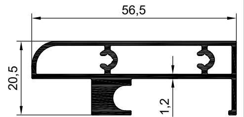
NO:7459 AĞIRLIK:756 gr/m
