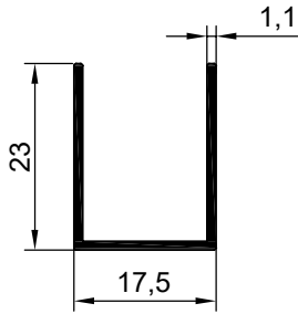
NO:6677 AĞIRLIK:182 gr/m
