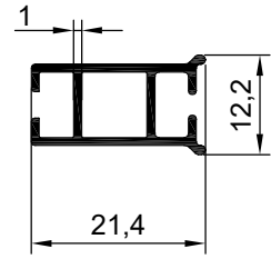
NO : 1987 AGIRLIK : 0.190 kg/m
