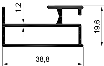
NO:6483 AĞIRLIK: 437 gr/m
