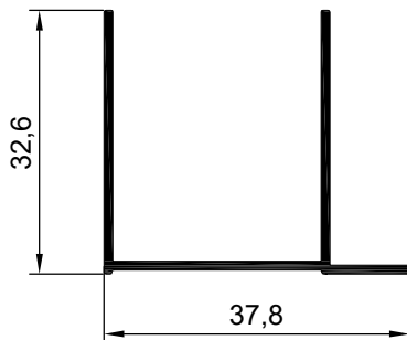
NO : 3045 AGIRLIK : 0.299 kg/m
