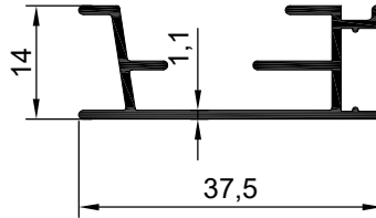
NO : 2482 AGIRLIK : 0.281 kg/m
