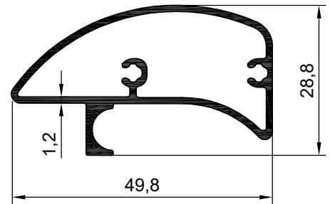
NO : 11874 AĞIRLIK : 0.549 kg/m
