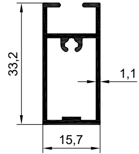
NO:6589 AĞIRLIK: 337 gr/m
