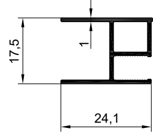
NO:7695 AĞIRLIK:220 gr/m
