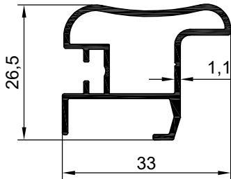
NO : 3038 AGIRLIK : 0.360 kg/m
