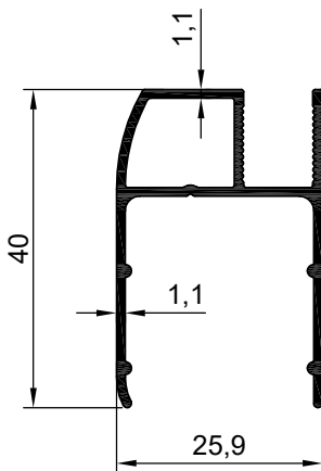
NO:7385 AĞIRLIK: 394 gr/m
