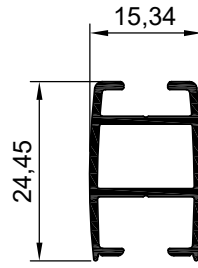
NO:7844 AĞIRLIK: 246 gr/m
