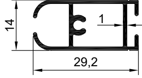
NO : 2478 AGIRLIK : 0.279 kg/m
