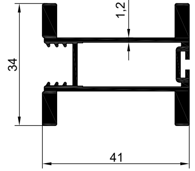
NO:6773 AĞIRLIK: 817 gr/m
