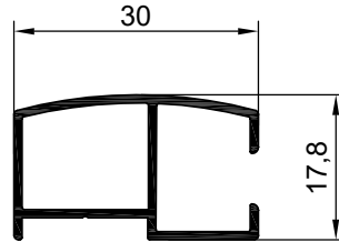
NO:7845 AĞIRLIK: 262 gr/m
