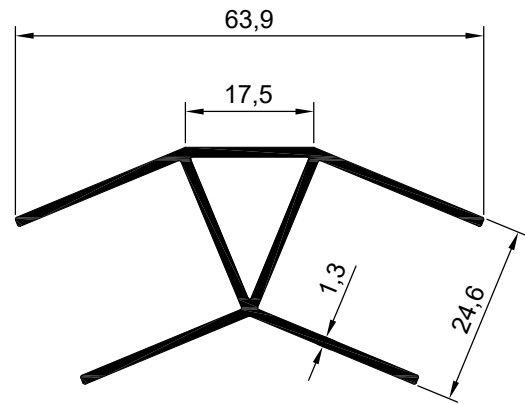
NO : 2142 AGIRLIK : 0.565 kg/m
