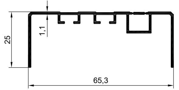
NO:7274 AĞIRLIK: 469 gr/m
