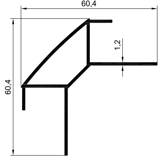
NO:6490 AĞIRLIK: 564 gr/m
