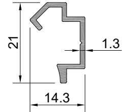
Profil No: W-546 Ağırlık : 152 gr/m
