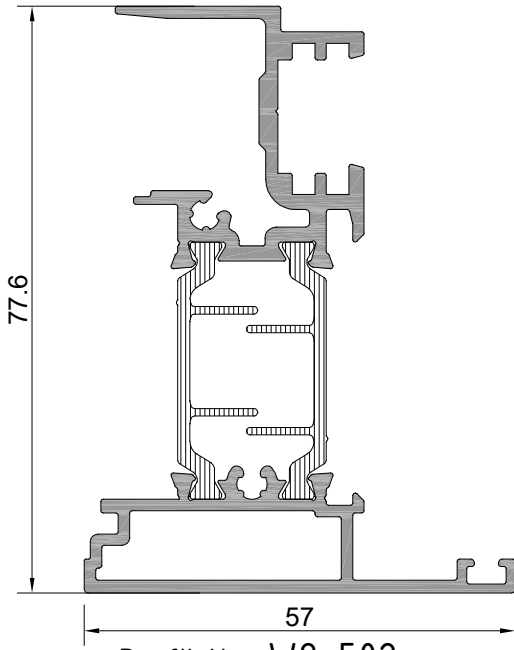
Profil No: W8-502
