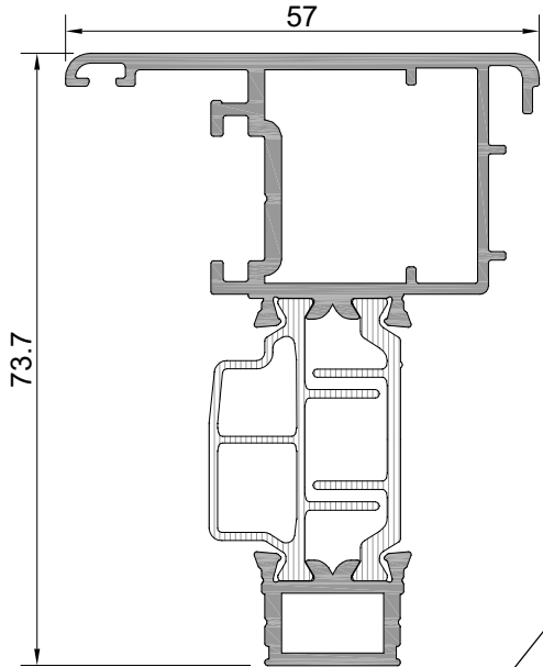
Profil No: W8-504
