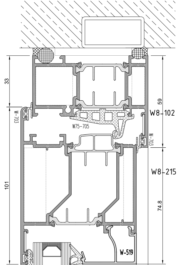
dışa açılım kapı outside opening door
