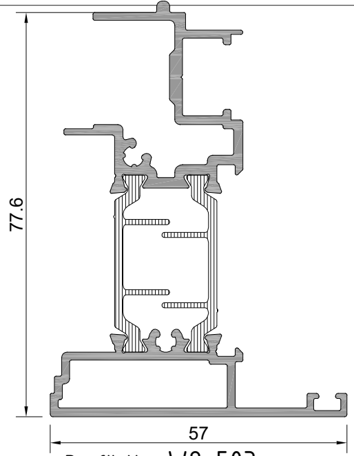
Profil No: W8-503
